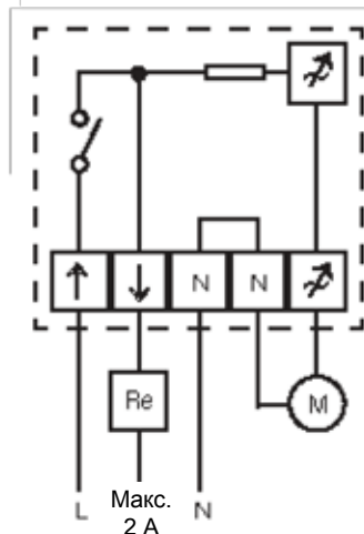
Схема соединений
